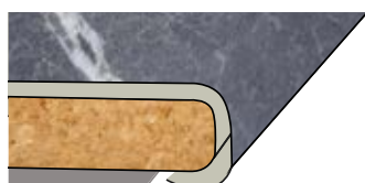
bordo postformato doppio raggio 8
