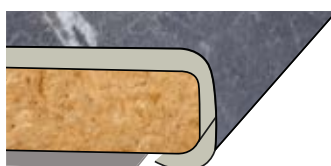
bordo postformato doppio raggio 4
