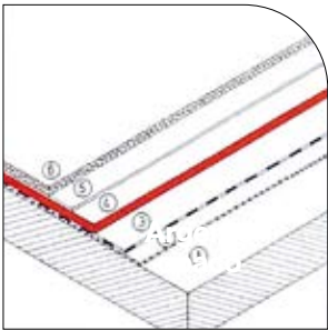
Isolamento di un tetto
